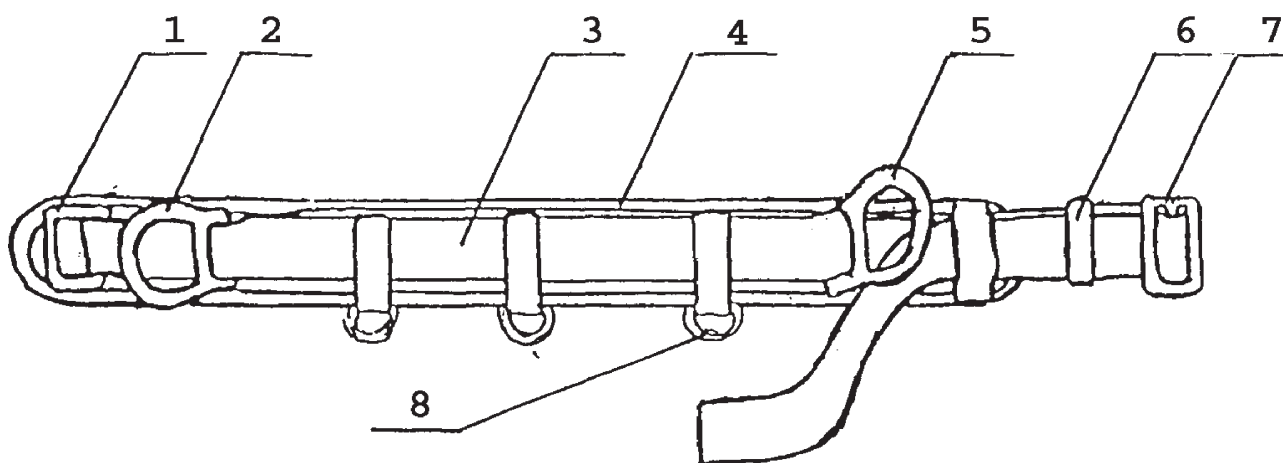
Рис. 1. Пояс предохранительный безлямочный:
