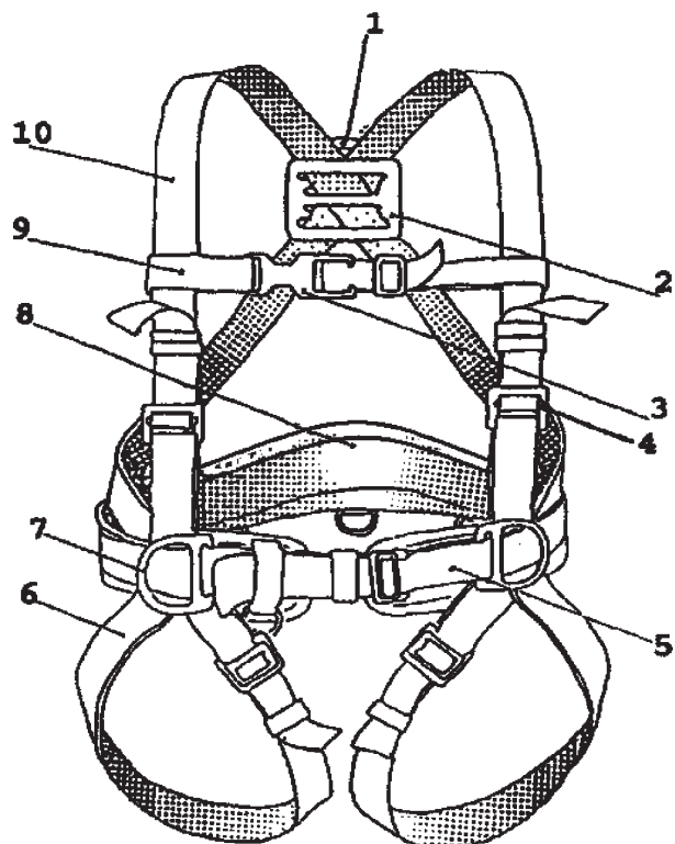
Рис. 2. Пояс предохранительный лямочный с наспинным и боковыми страховочными узлами 1ПЛ-К:
